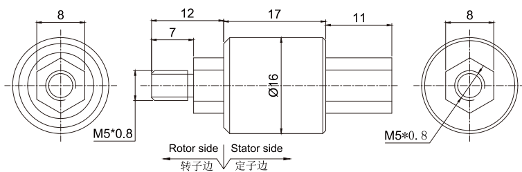
MW-A1M5 尺寸图
