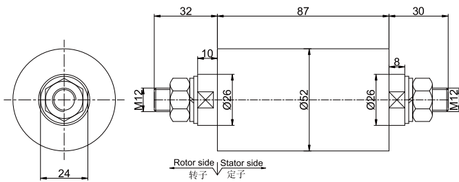
MW5045-P01250 尺寸图
