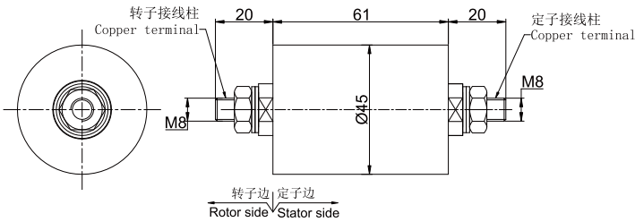
MW5045-P01200 尺寸图
