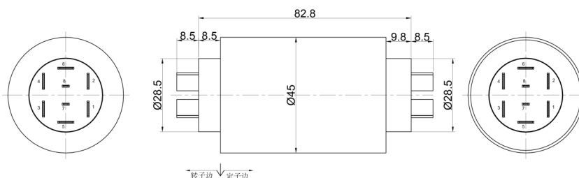
MW4045-P0630-S02 尺寸图
