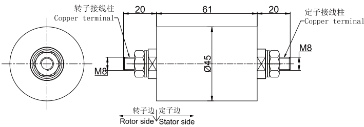
MW5045-P01150 尺寸图
