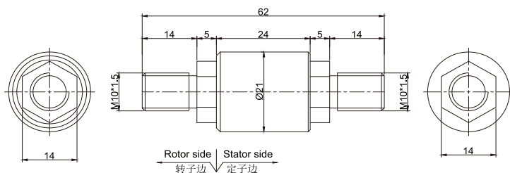
MW-A1H25 尺寸图
