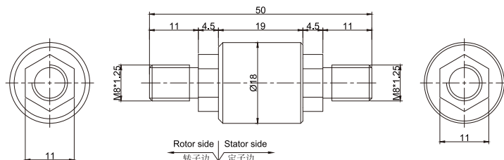
MW-A1M5 尺寸图
