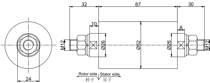
MW5045-P01250 尺寸图
